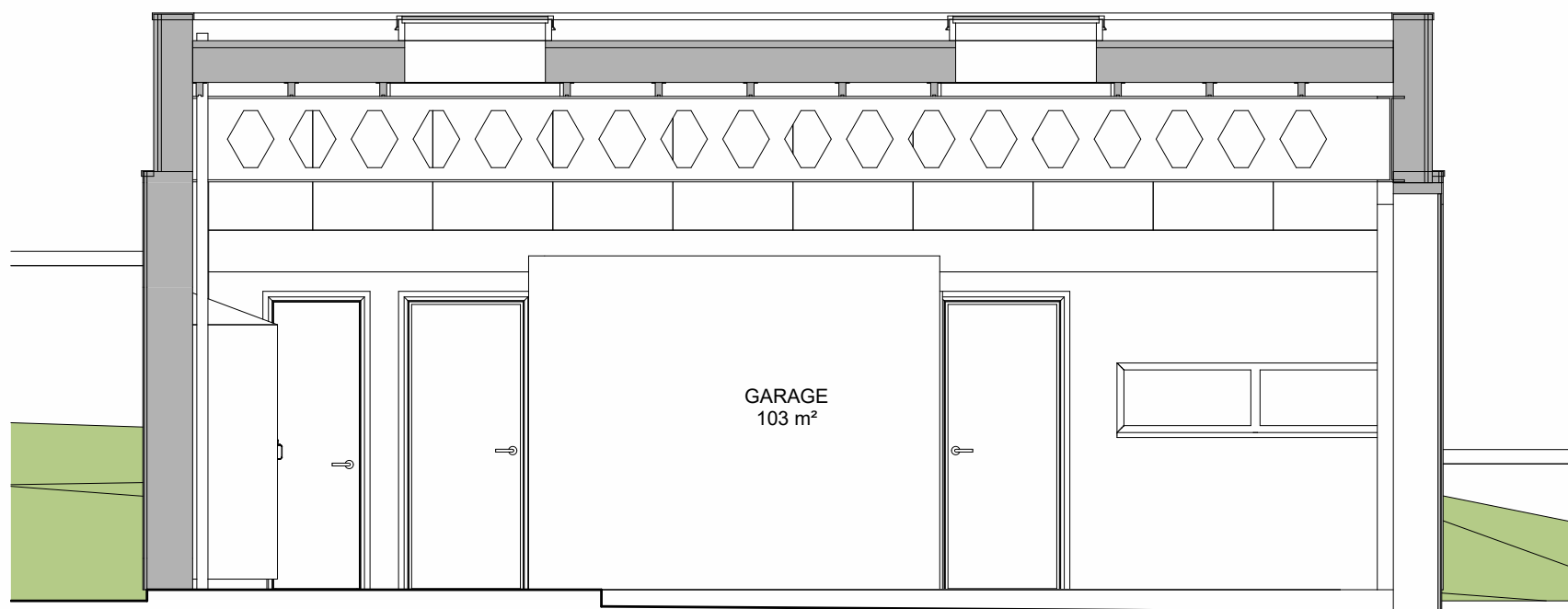
⑤ Section 1 1 : 50
