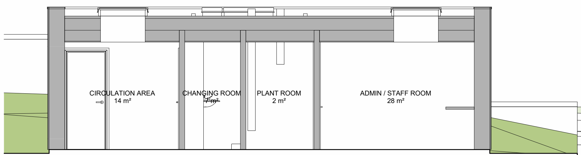
⑦ Section 3 1 : 50
